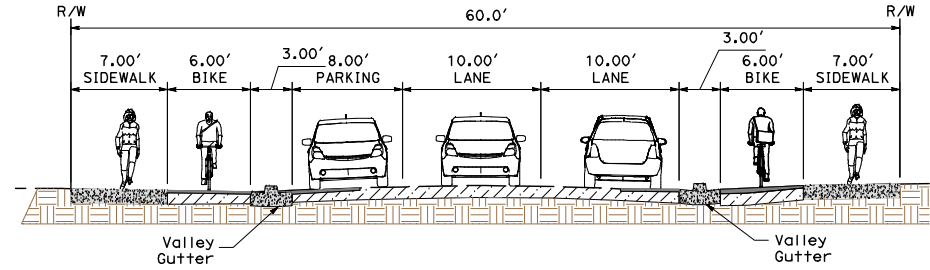
SECTION D-D SCALE: NO SCALE
