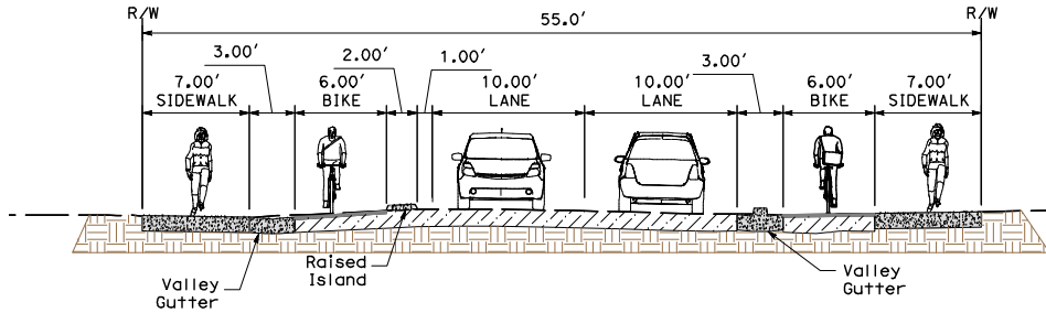
SECTION B-B SCALE: NO SCALE
