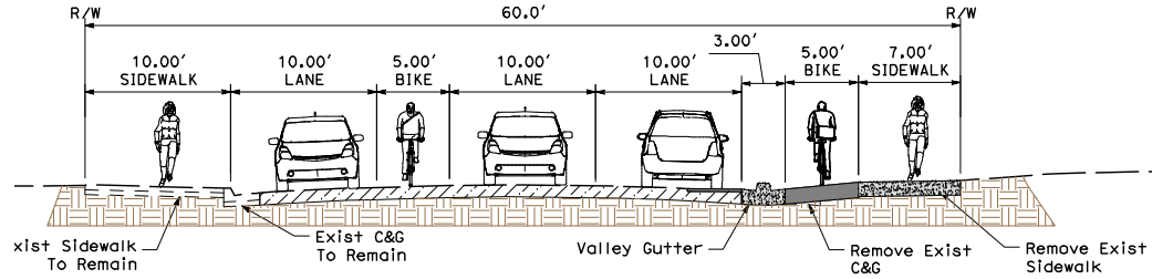
SECTION A-A SCALE: NO SCALE
